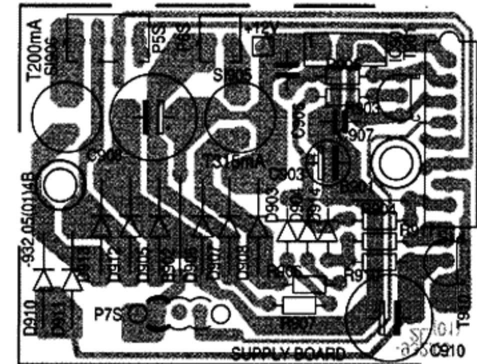
Spannungsversorgungsplatte / Supply Board
