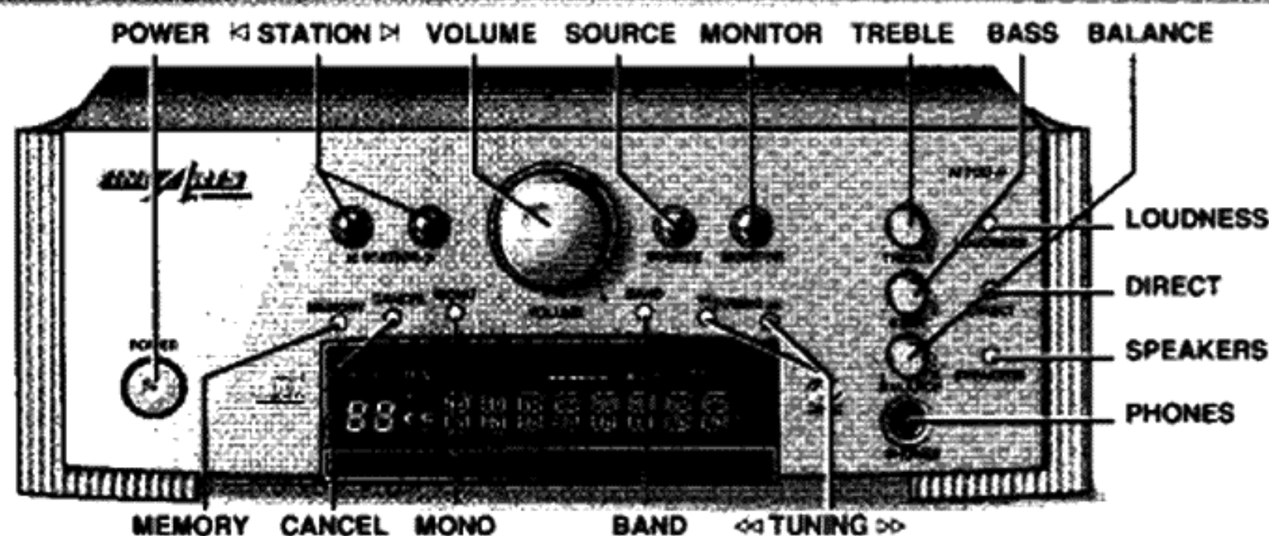
Vorderseite des Receivers
