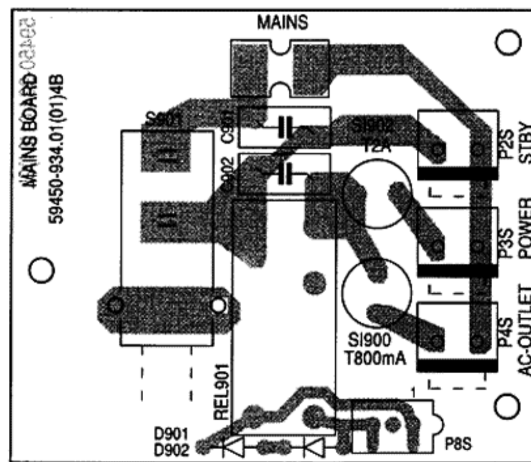
Netzteilplatte / Mains Board
