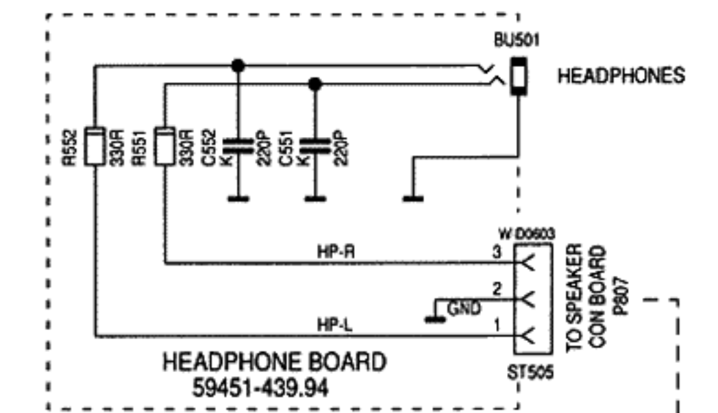
Kopfhörerbuchsenplatte Headphone Socket Board
