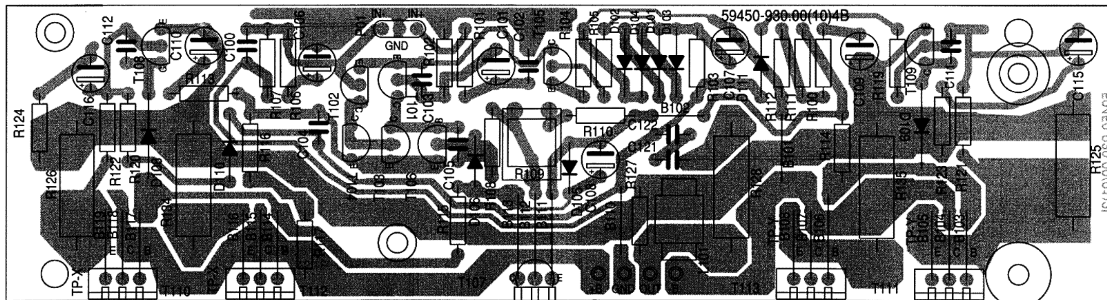
Verstärkerplatte / Amplifier Board
