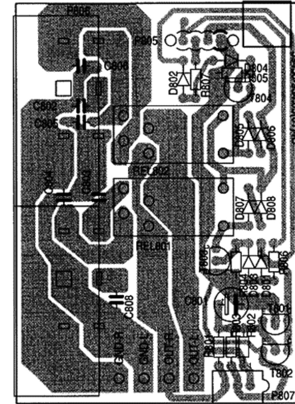
NF-Ausgangsplatte / AF Output Board
